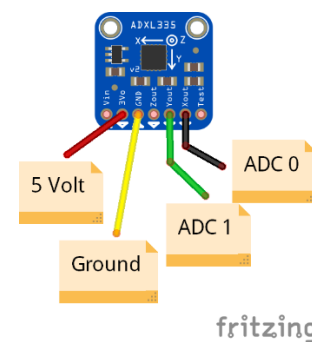
Gambar 2. Rangkaian Sensor ADXL335.
