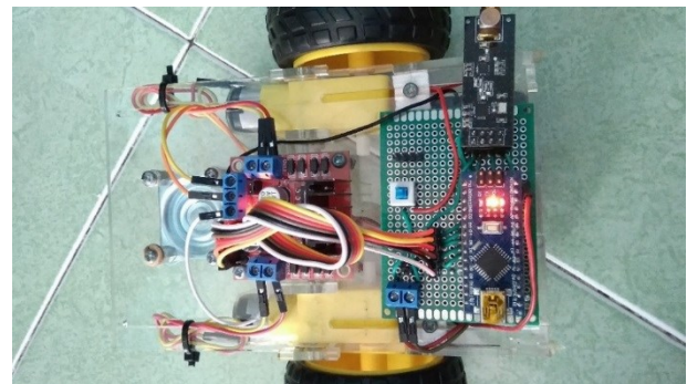
Gambar 16. Tahap percobaan rangkaian Mobile robot .
