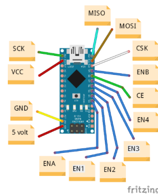
Gambar 3. Rangkaian Arduino Nano.
